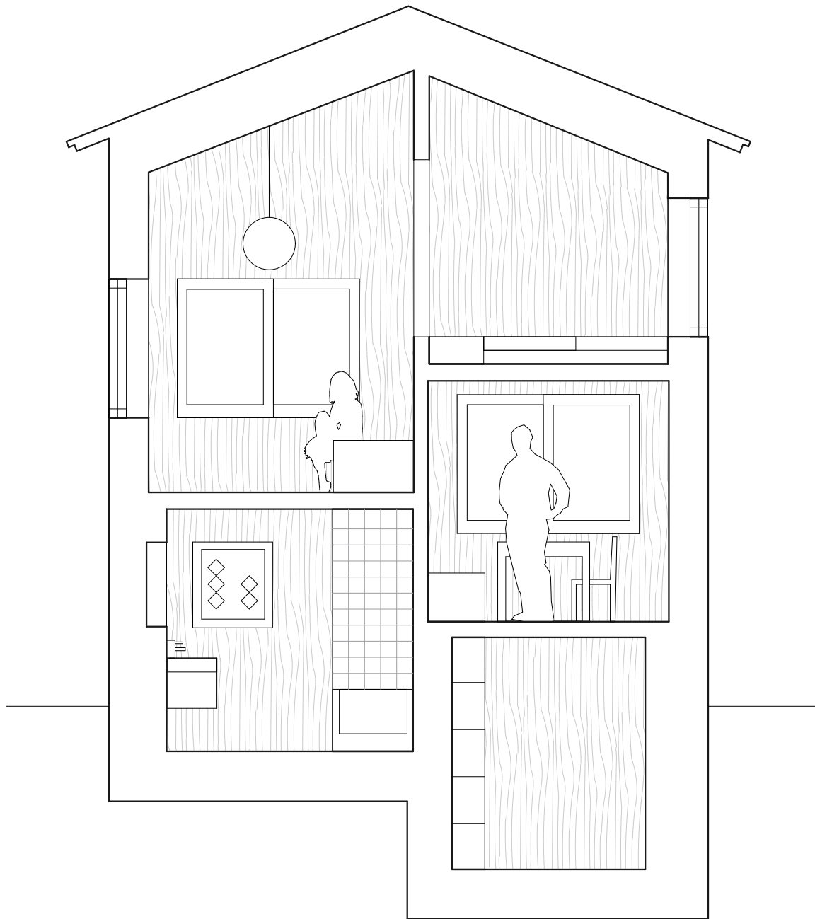
coupe 1:50
