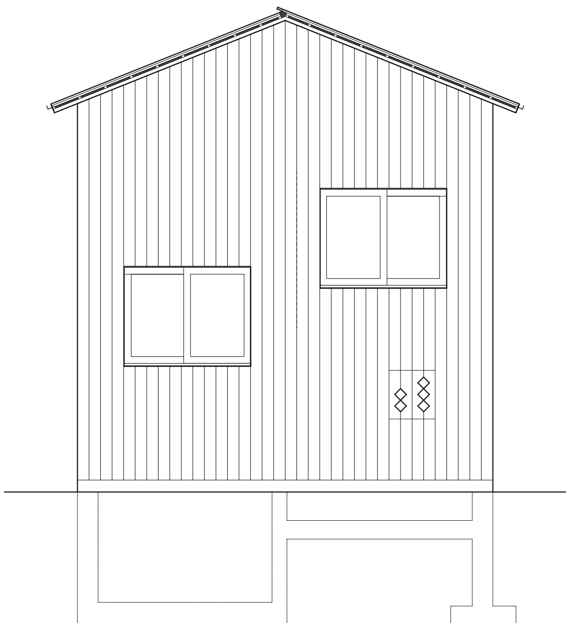
façade est 1:50
