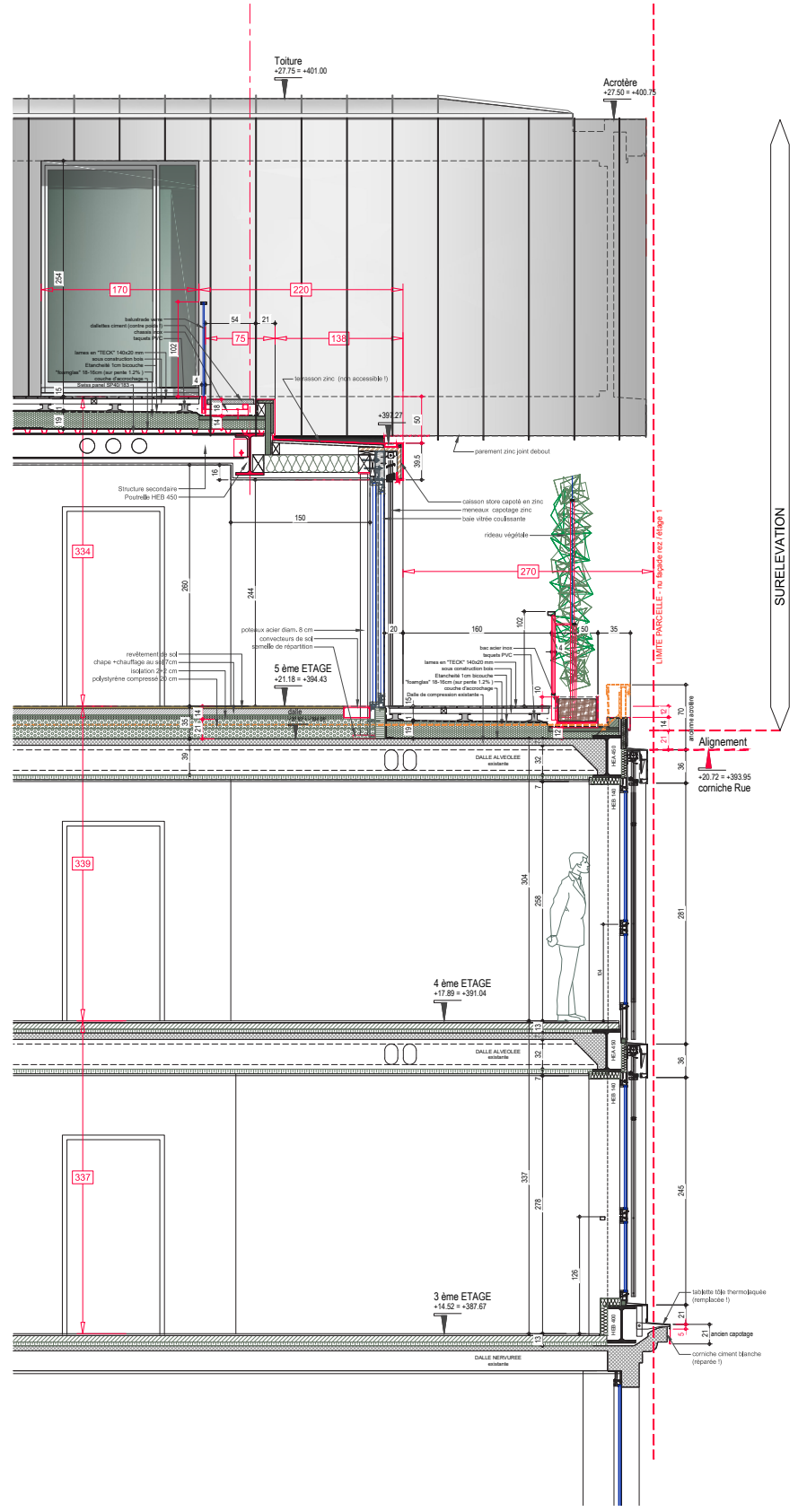
COUPE E
