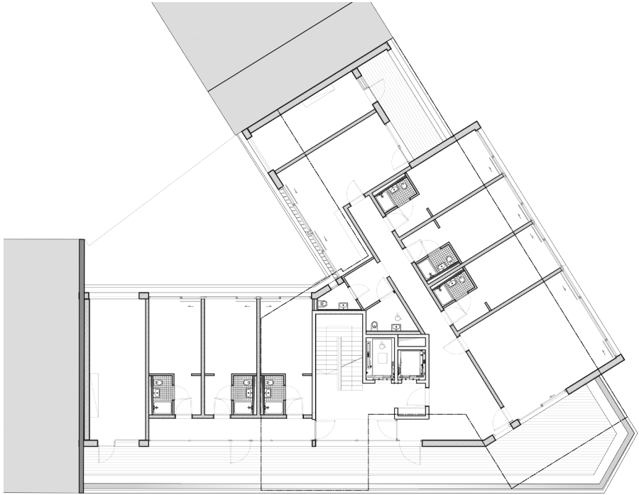
PLAN ETAGE 6
