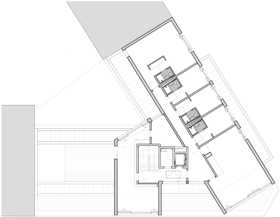
PLAN ETAGE 7
