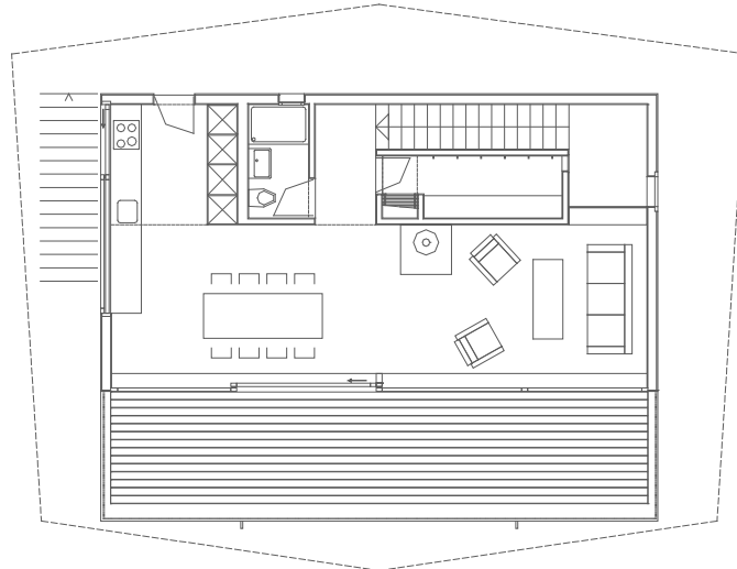
niveau 1 séjour
