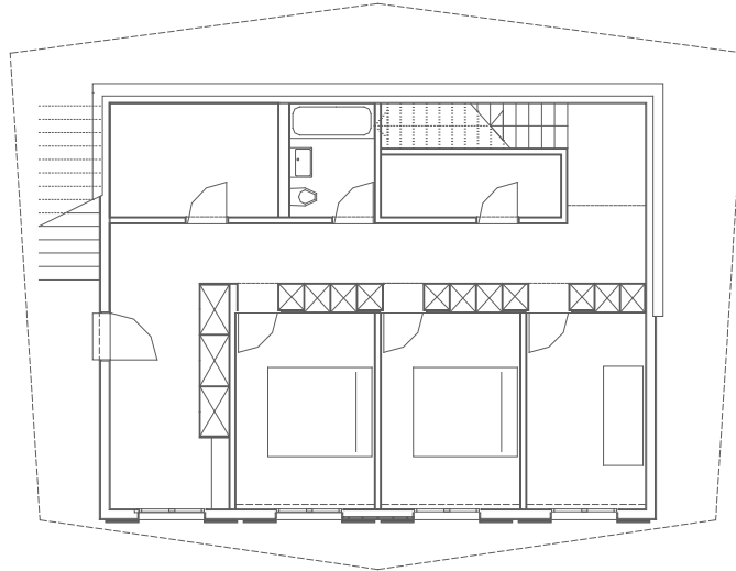
niveau 0 chambres
