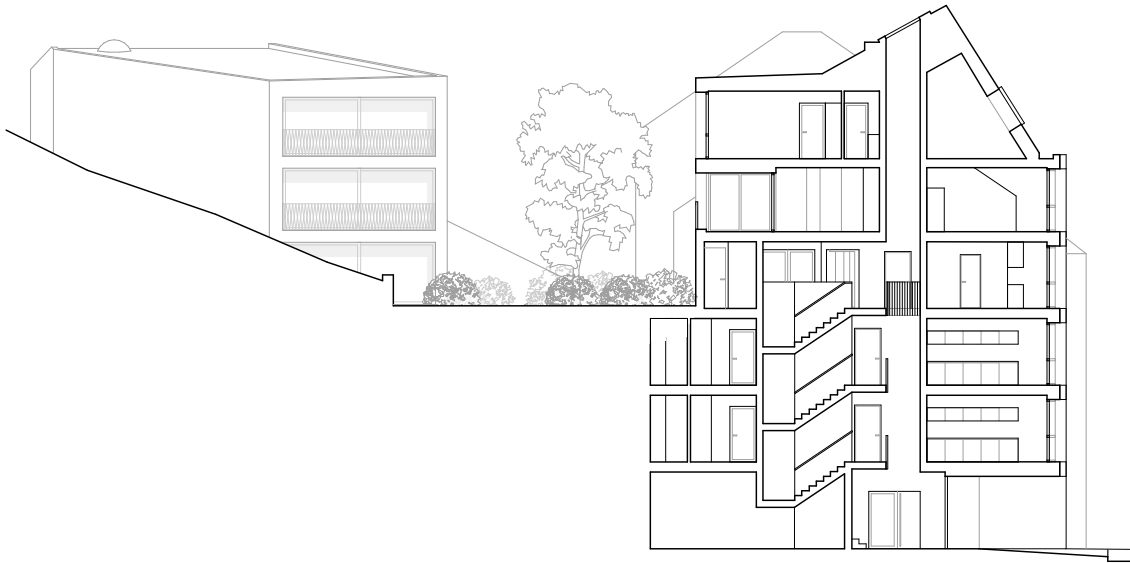
COUPE LONGITUDINALE
