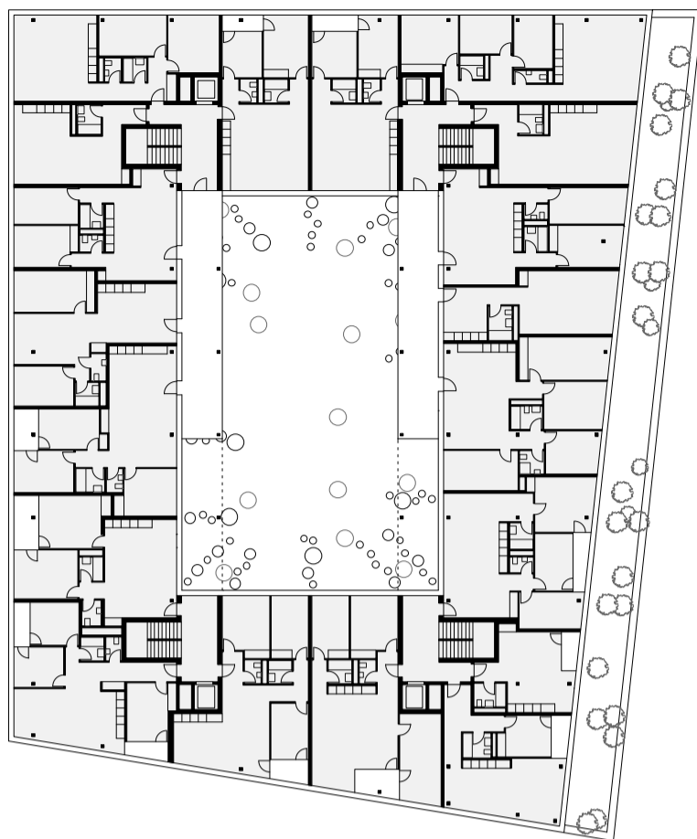
Plan étage pair 1:500
