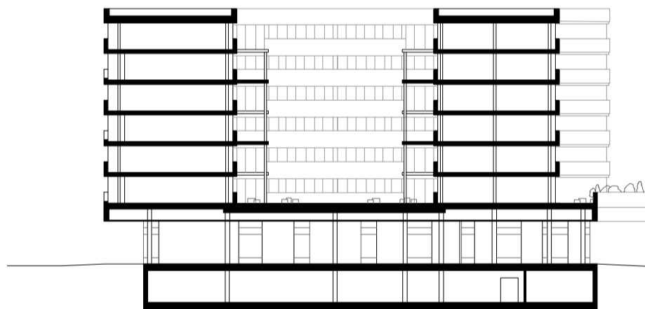
Coupe transversale 1:500
