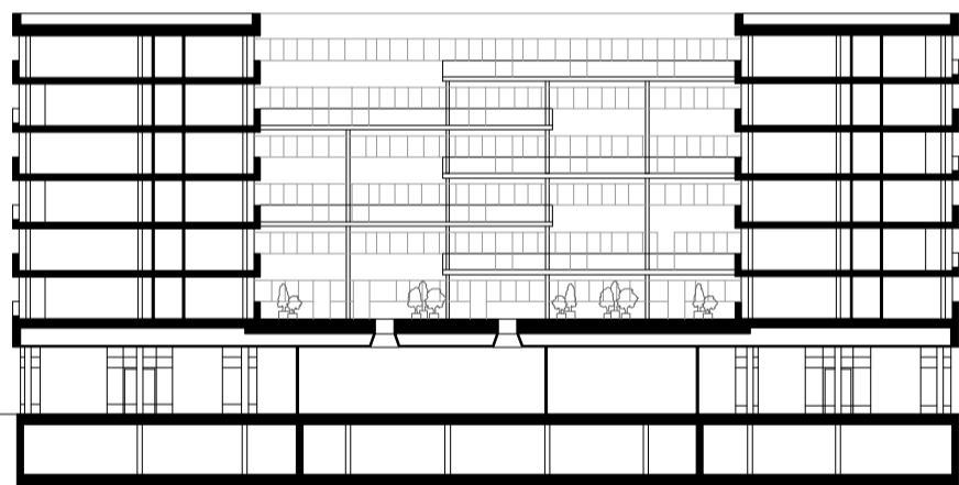
Coupe longitudinale 1:500
