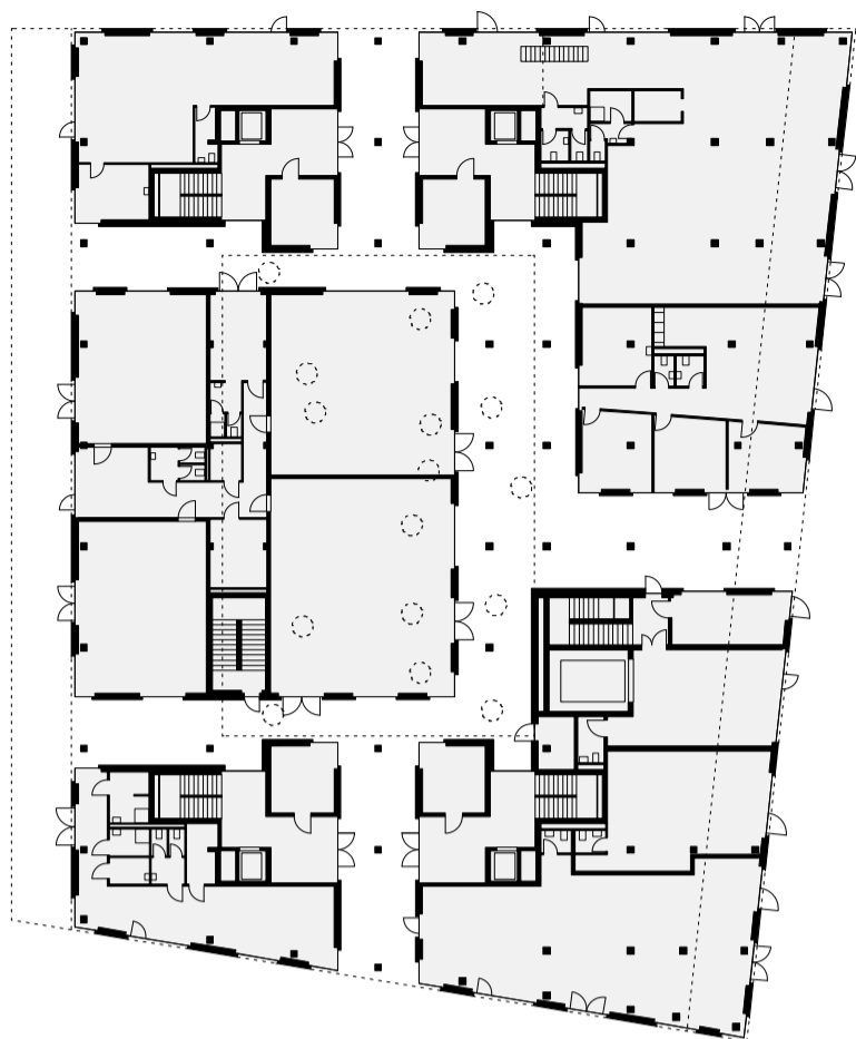
Plan rez-de-chaussée 1:500
