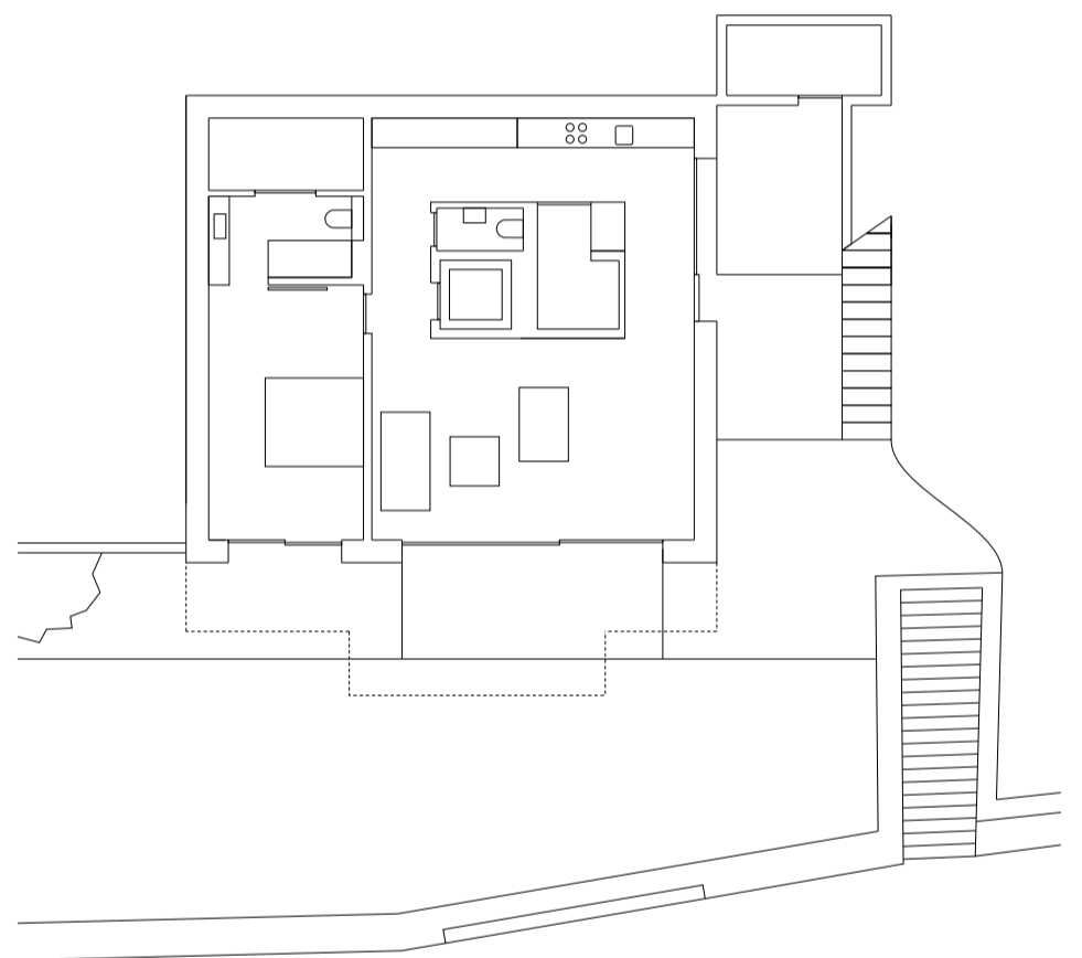
NIVEAU -1
