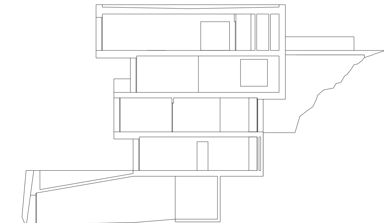
COUPE TRANSVERSALE
