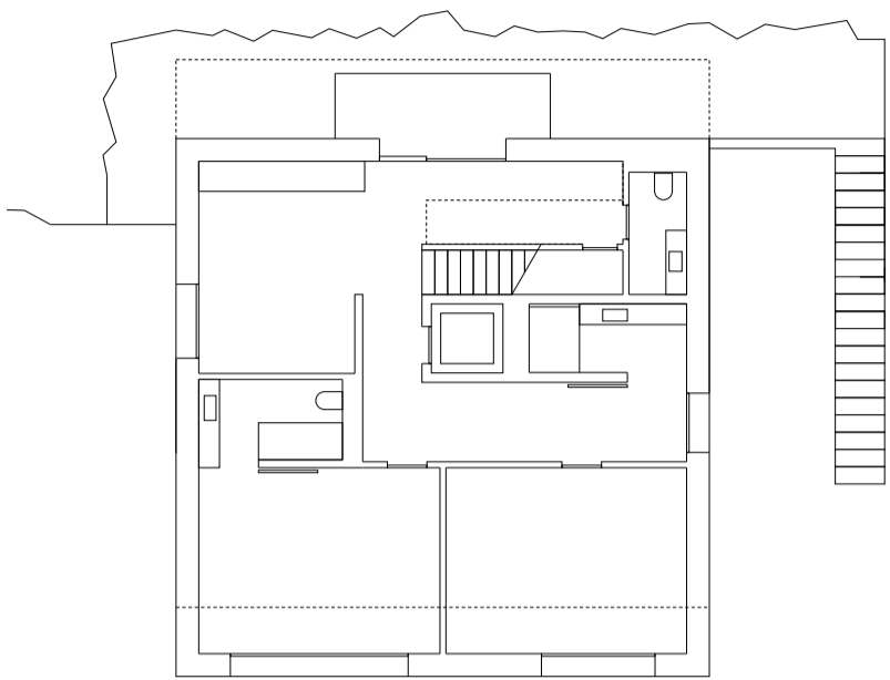
NIVEAU 0
