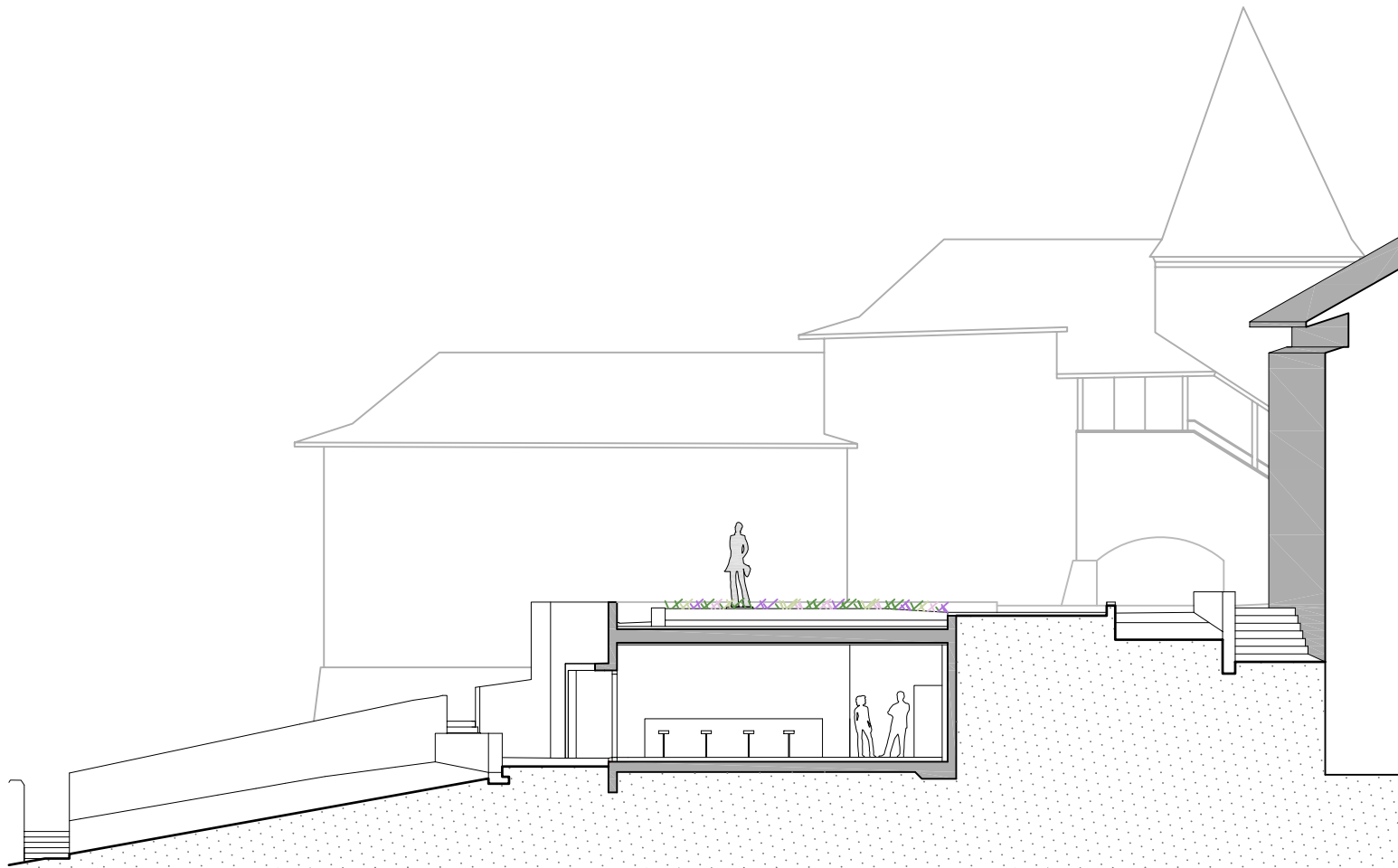
coupe transversale
