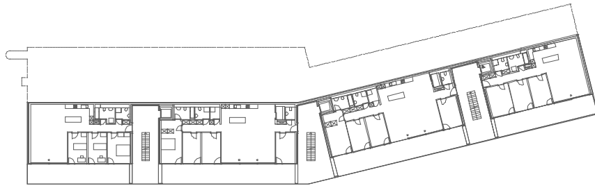
niveaux 0 et 1
