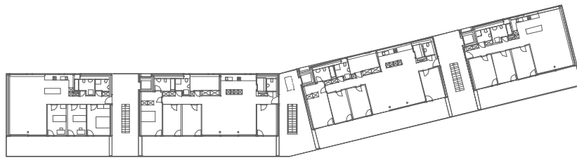
niveaux 5
