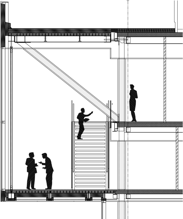
Coupe transversale du porte-à-faux
