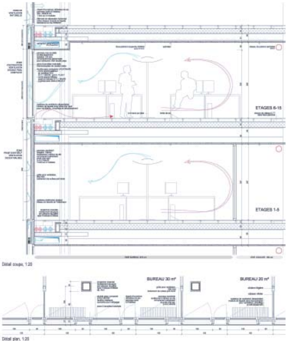
Détails de principe de façade
