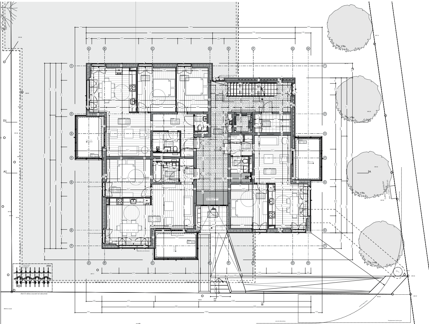
REZ-DE-CHAUSSEE
