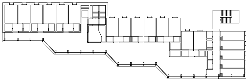
plan du 1 er étage
