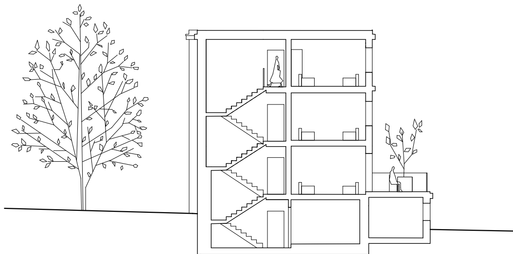
COUPE BB
