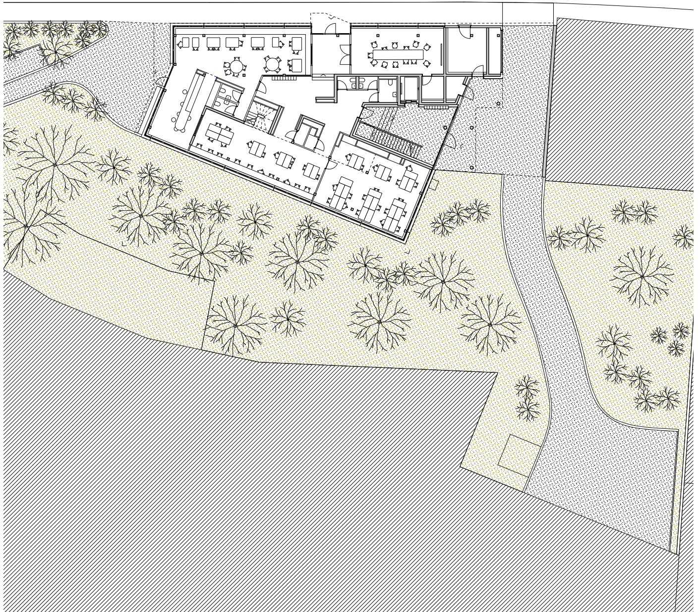
Plan Rez-de-chaussée
