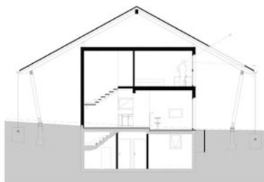
COUPE TRANSVERSALE
