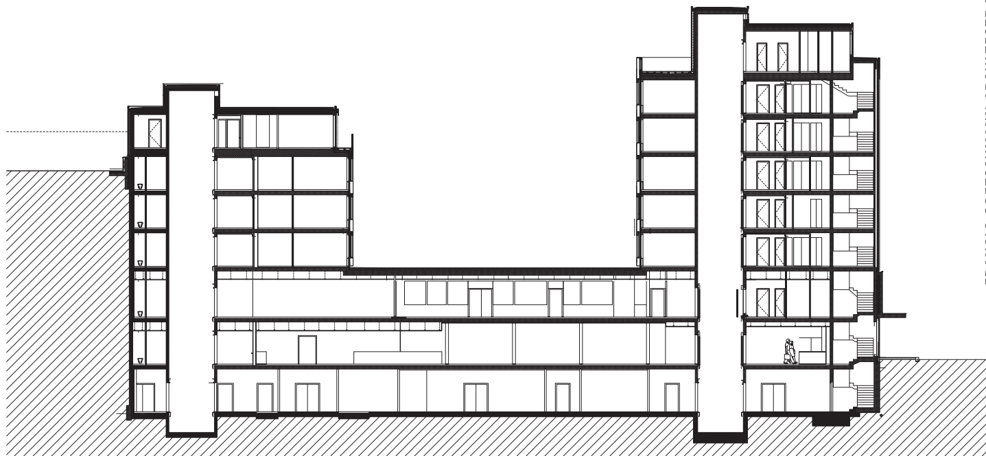
COUPE TRANSVERSALE
