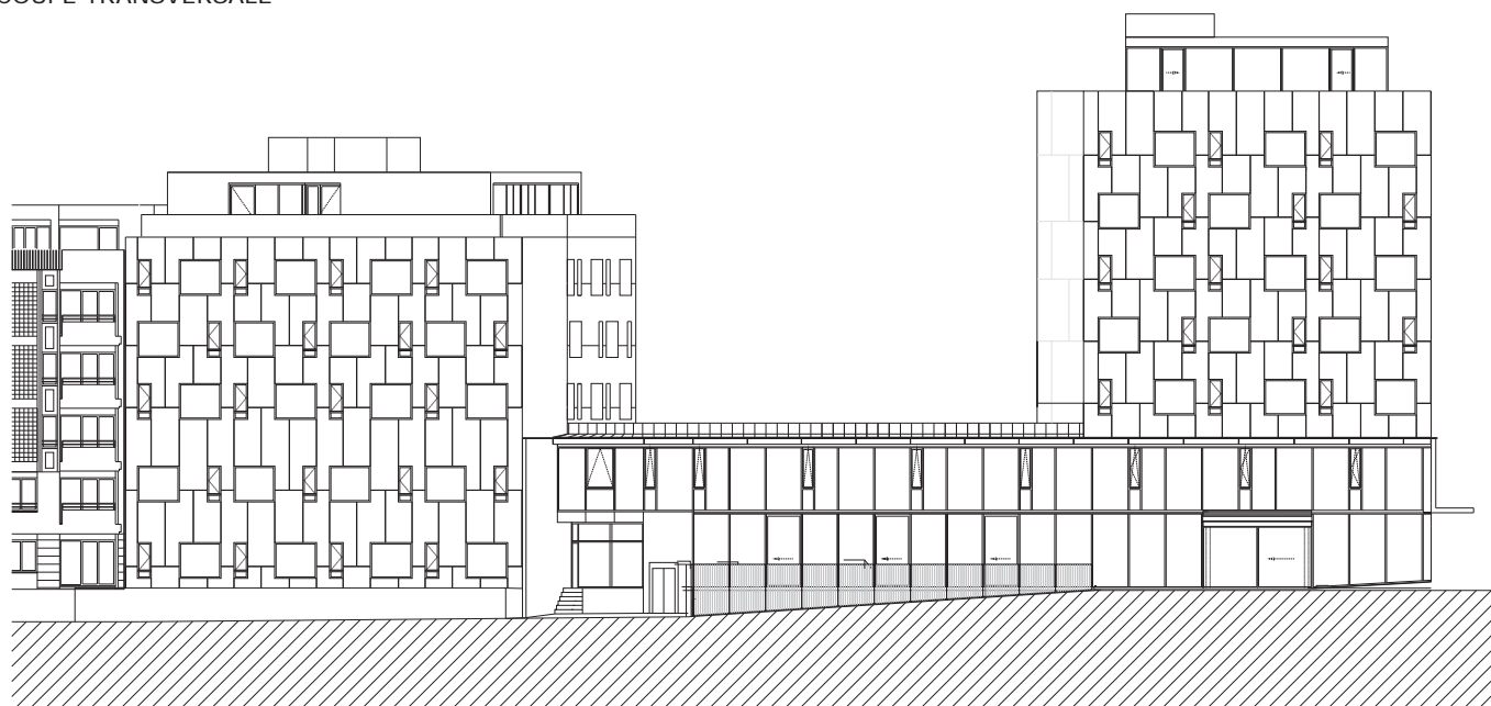
ELEVATION SUD-EST
