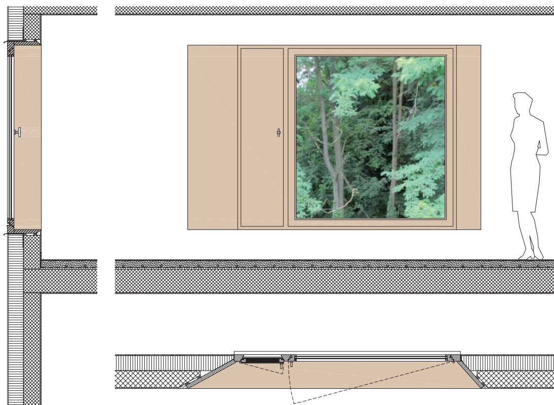
Plan, coupe et élévation d'une fenêtre type
