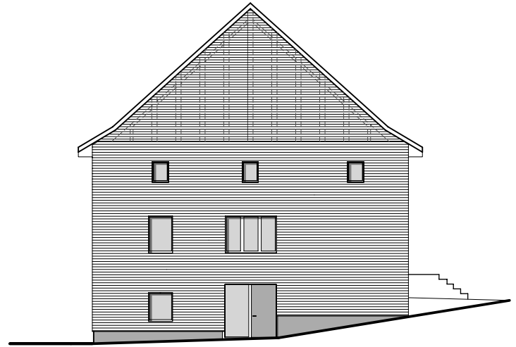
FACADE EST
