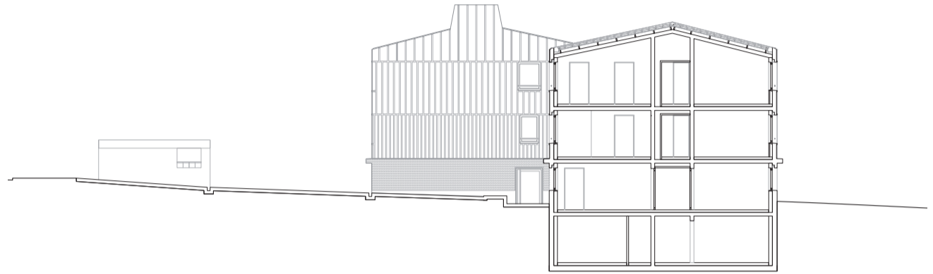
Coupe 03
