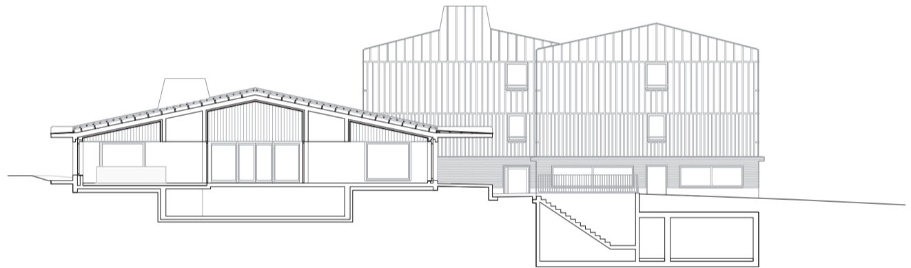
Coupe 04
