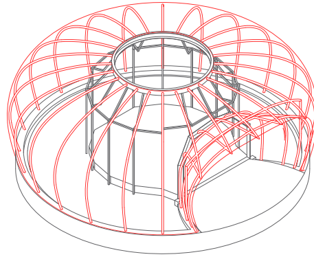
2. Mise en place des cintres réticulés, ferrailage et gunnitage
