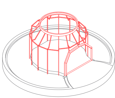
1. Construction du radier, mise en place de la sous-construction et de l'anneau sommital
