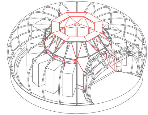
4. Pose du bardage intérieur et sommital en inox
