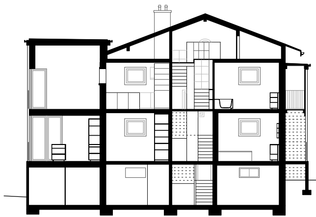
Coupe transversale 1:200
