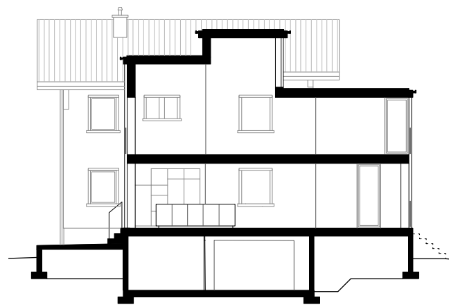
Coupe longitudinale 1:200
