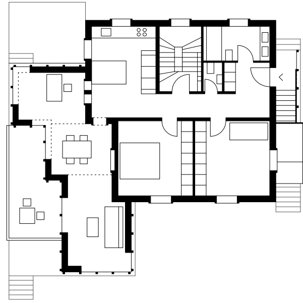
Plan premier étage 1:200
