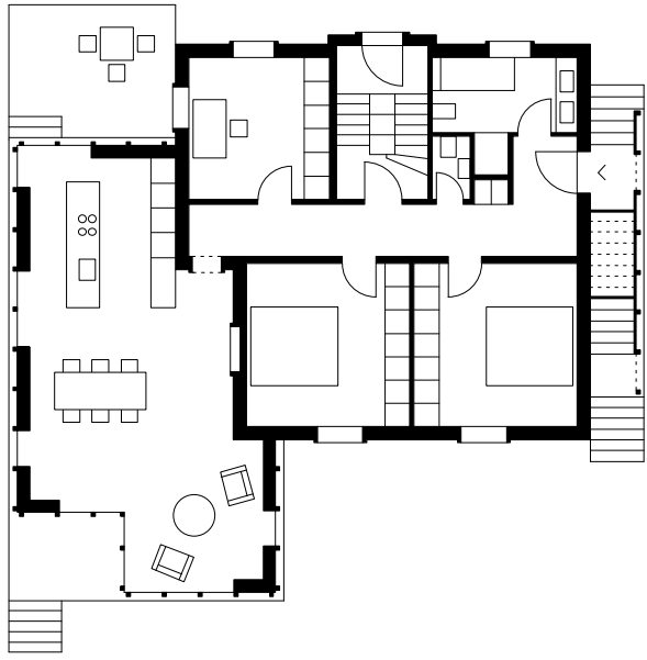
Plan rez-de-chaussée 1:200
