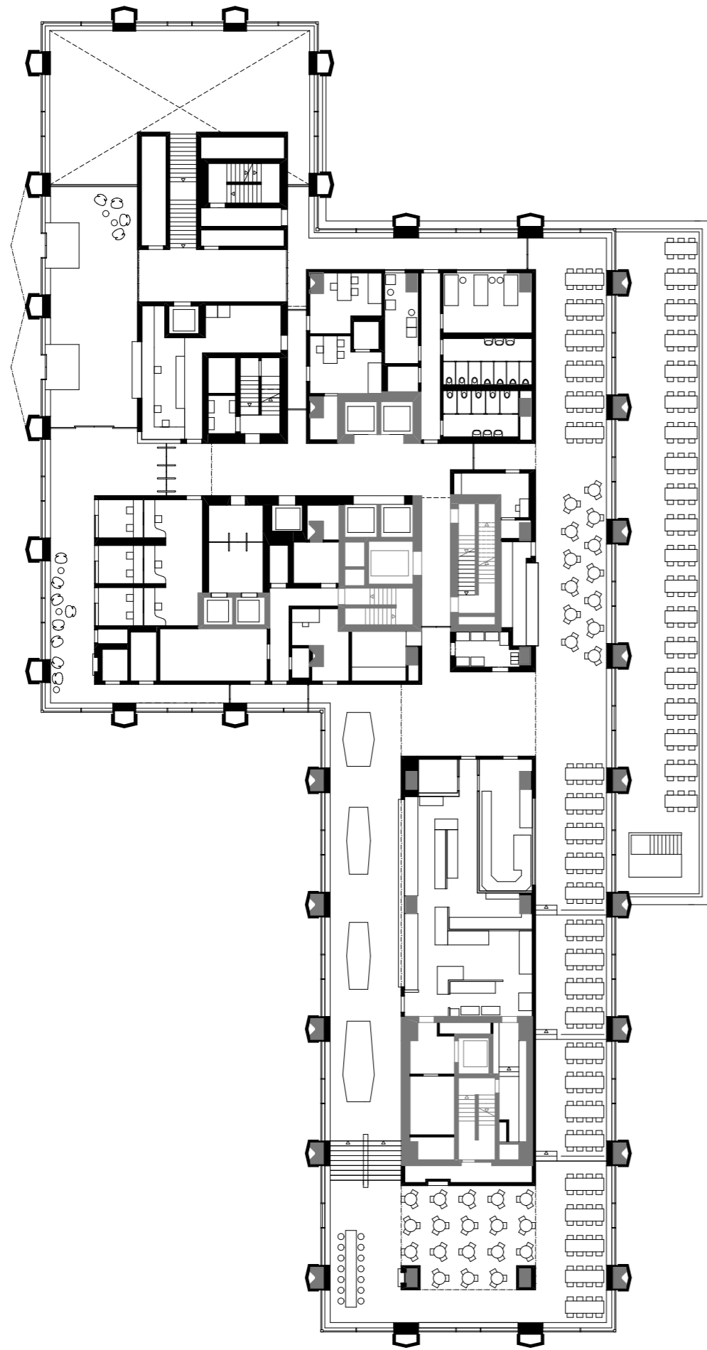
Rez-de-chaussée supérieur
