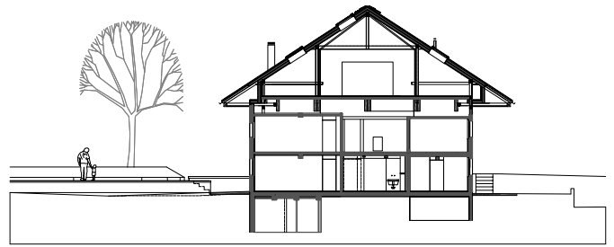
coupe B
