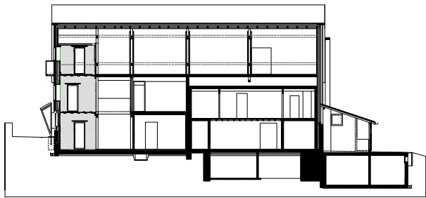
coupe A
