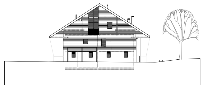
façade Sud
