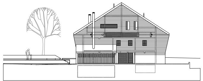
façade Nord
