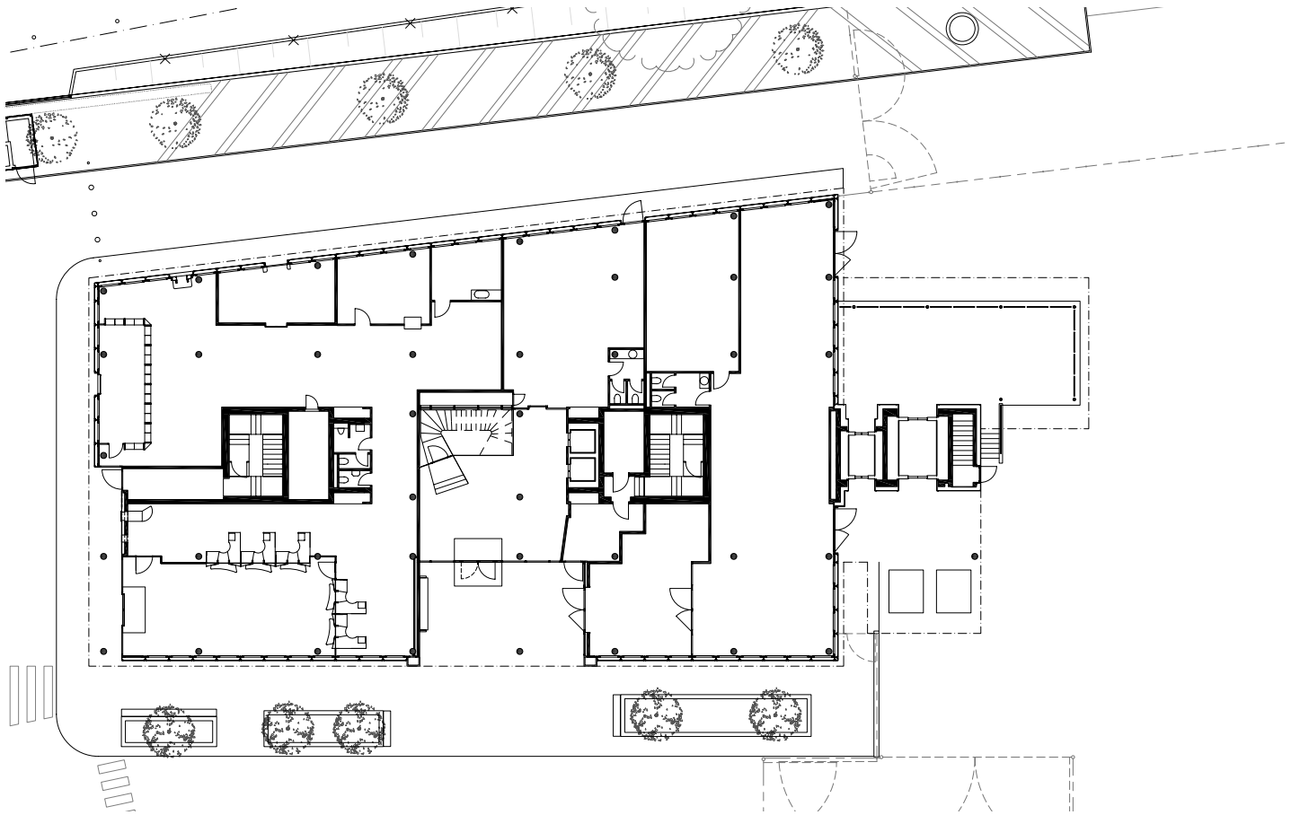
PLAN REZ-DE-CHAUSSEE
