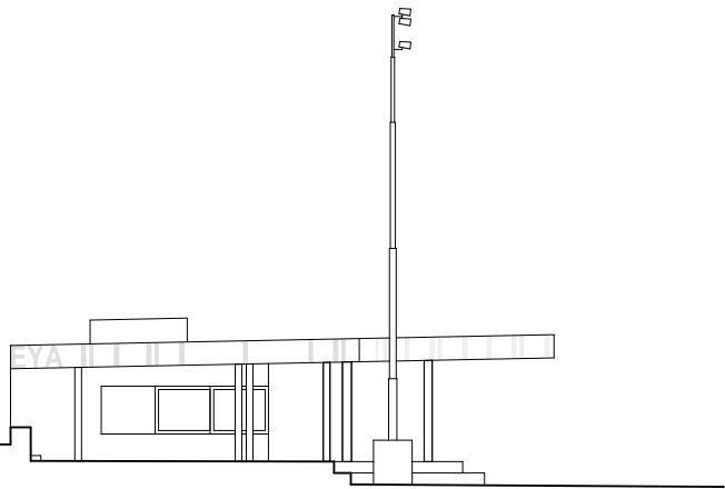
façade sud
