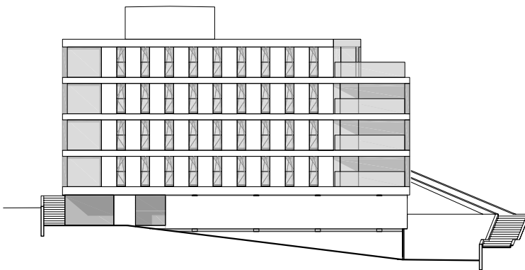
façade sud
