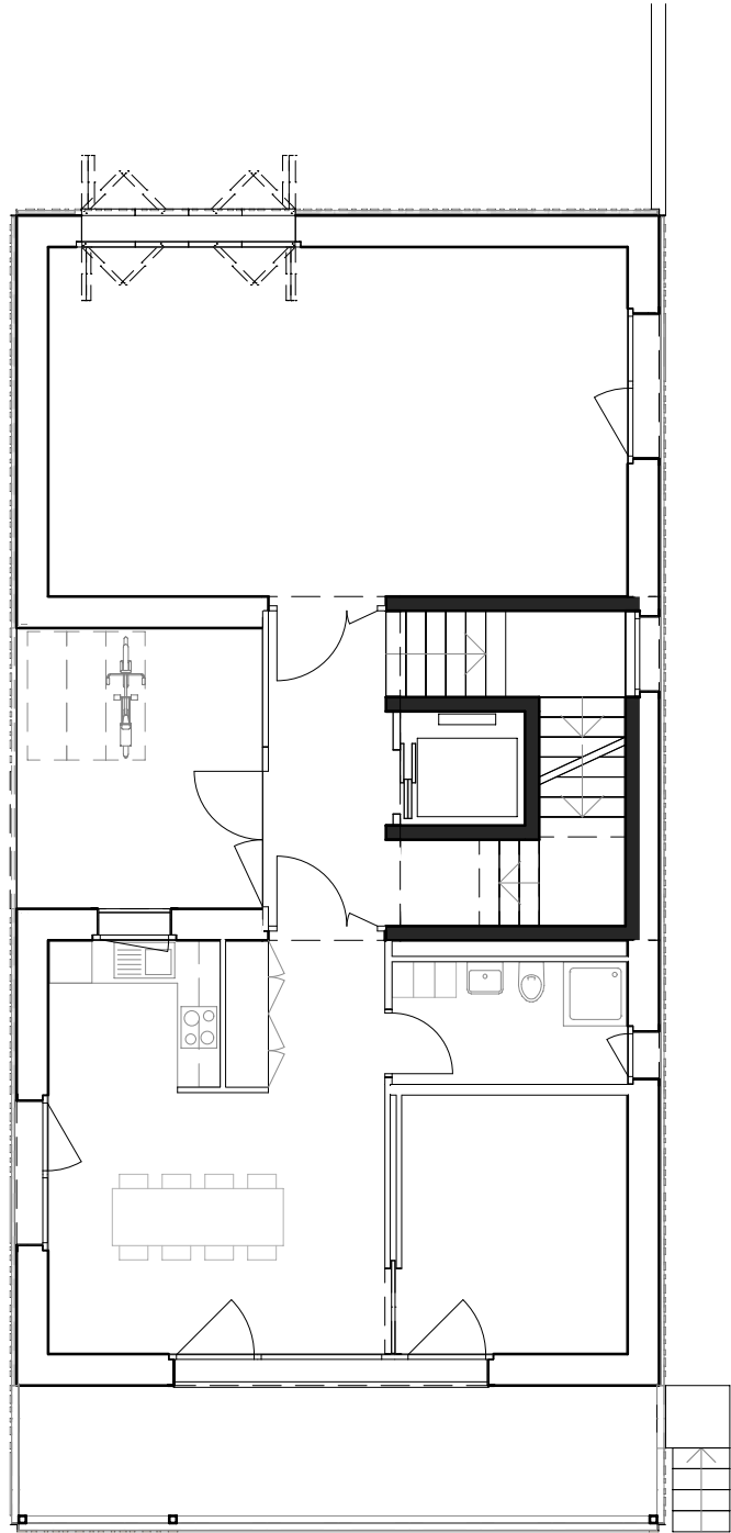
Plan du rez-de-chaussée
