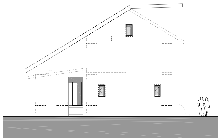
Façade NE
