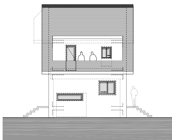
Façade SE
