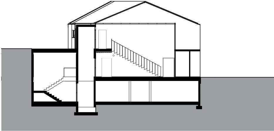
Coupe 1:250
