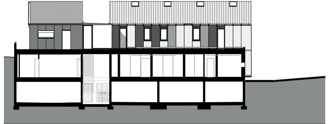
Façade Nord 1:250
