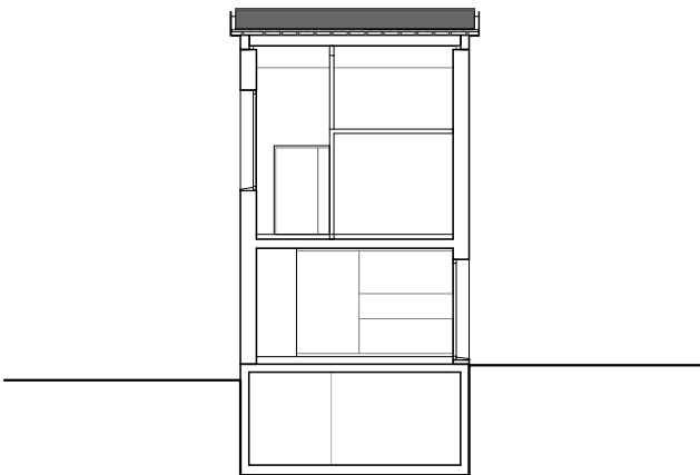
Coupe transversale
