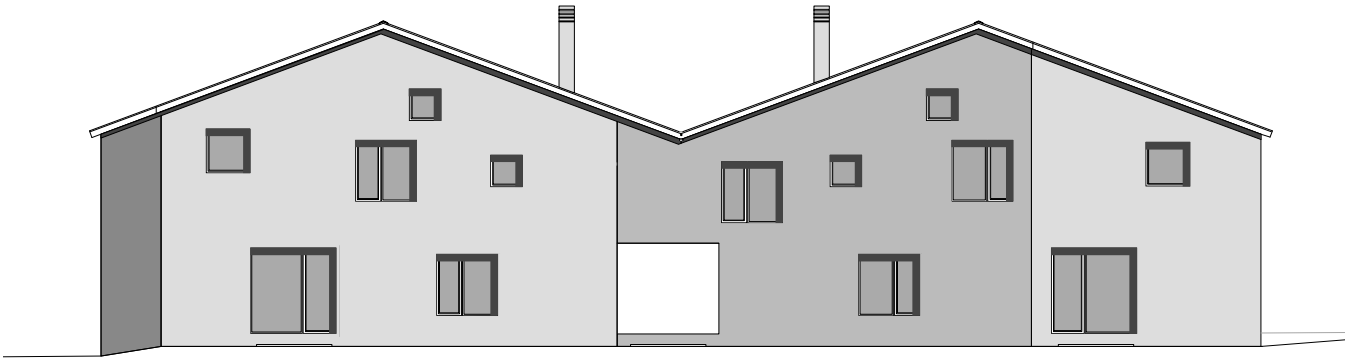
Élévation sud
