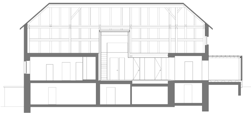
Coupe transversale
