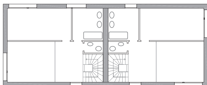
Plan du 1er étage 1:200
