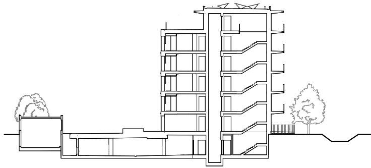
Coupe A-A 0 5.5 11 27.5m
