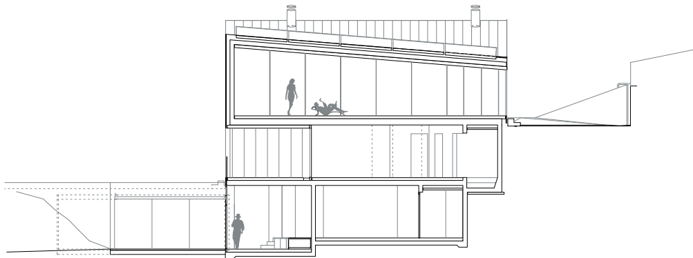
Coupe B
