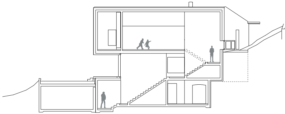
Coupe A
