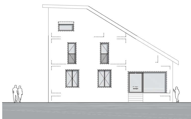
Façade SO
