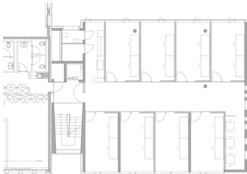
PLAN NIVEAUX 1-2-3-4
