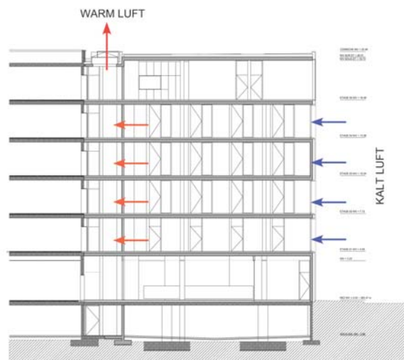
COUPE LONGITUDINALE – CONCEPT DE VENTILATION NATURELLE
