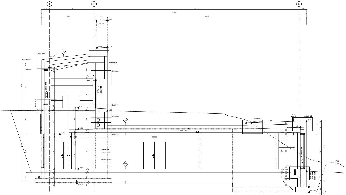
coupe longitudinale
