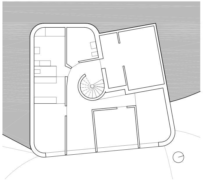
Rez inférieur
