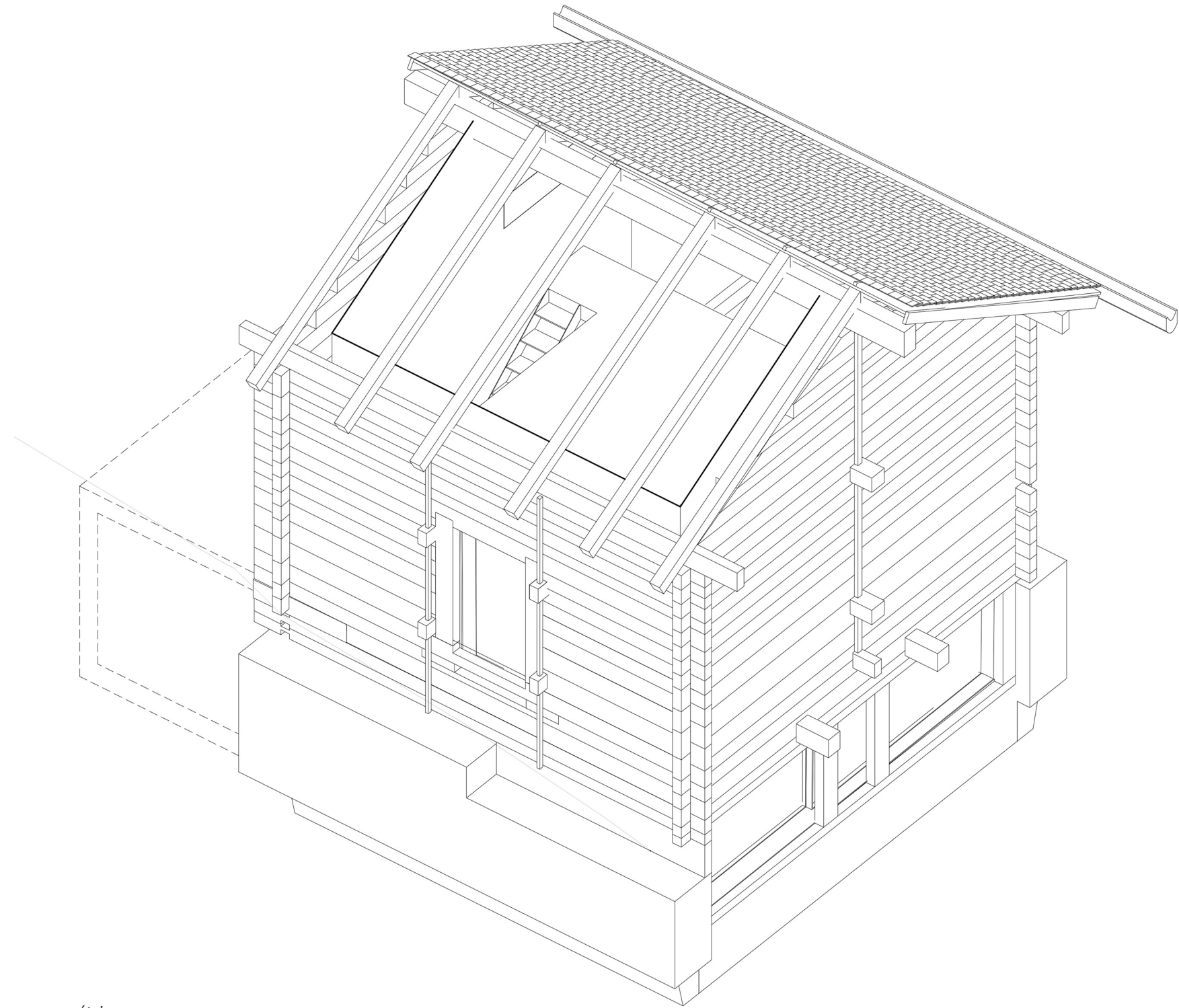
axonométrie
