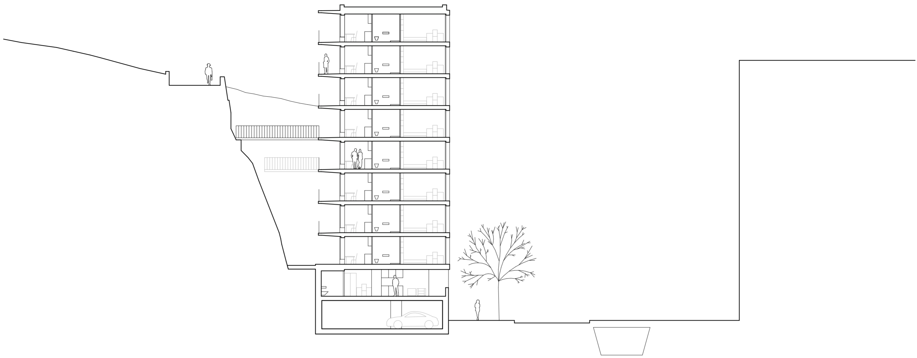
Coupe transversale
