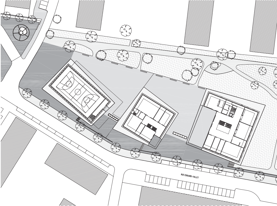
Plan des rez-de-chaussée
