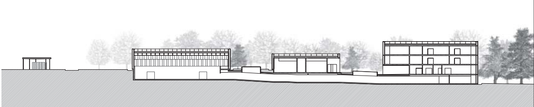
Coupe longitudinale sur le passage souterrain
