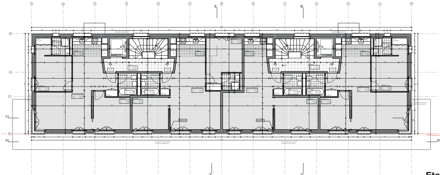
Etage 1
