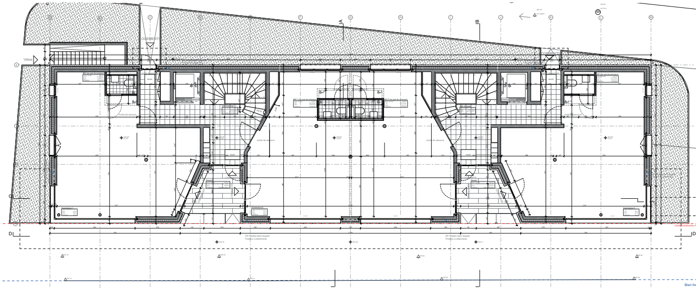
REZ-DE-CHAUSSEE
