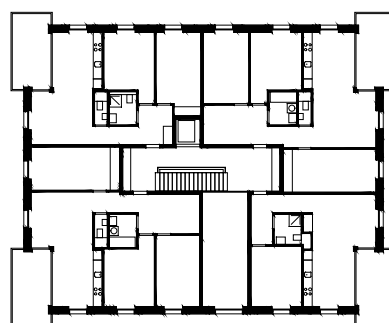
A28 Plan 2eme étage 1/500 0 5m
