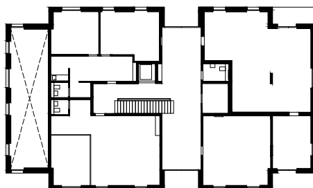
A24 + A25 Plan Rez Supérieur 1/500 0 5m
