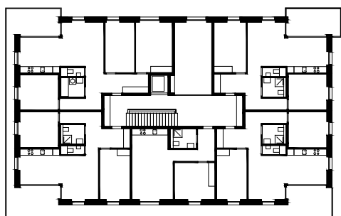
A24 + A25 Plan 1er étage 1/500 0 5m
