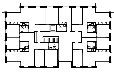
A24 + A25 Plan 2eme étage 1/500 0 5m
