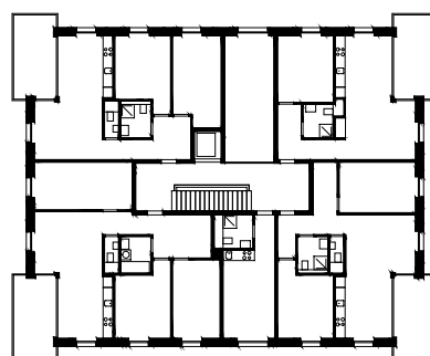
A28 Plan 3eme étage 1/500 0 5m
