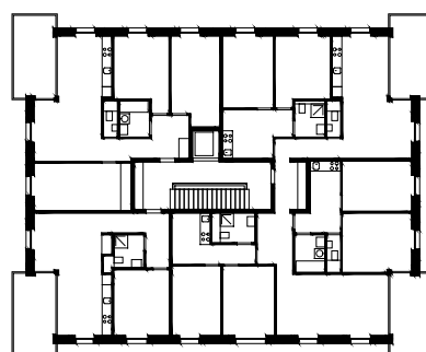
A28 Plan 1er étage 1/500 0 5m
