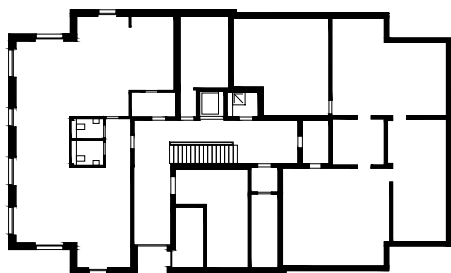
A24 + A25 Plan Rez Intérieur 1/500 0 5m
