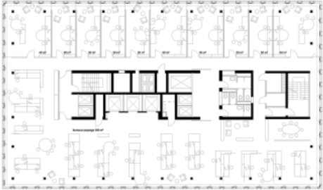
Plan d'un niveau type
