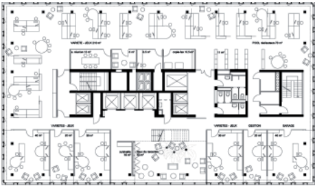
Plan d'un niveau avec patio
