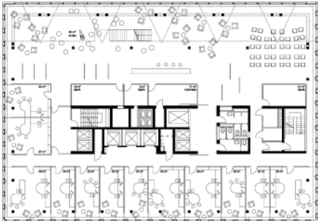
Plan du dernier niveau
