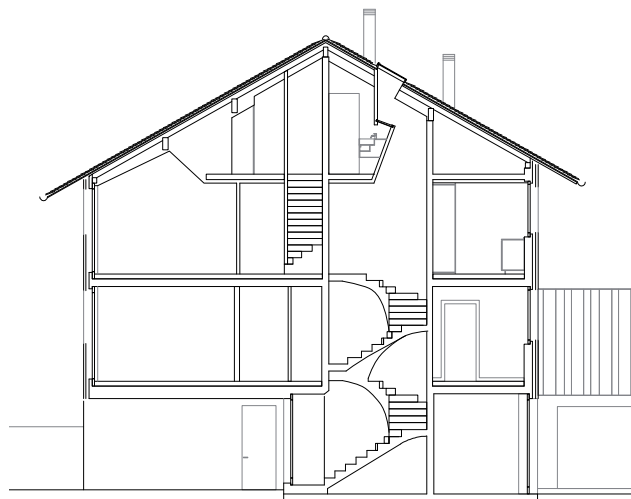
coupe
