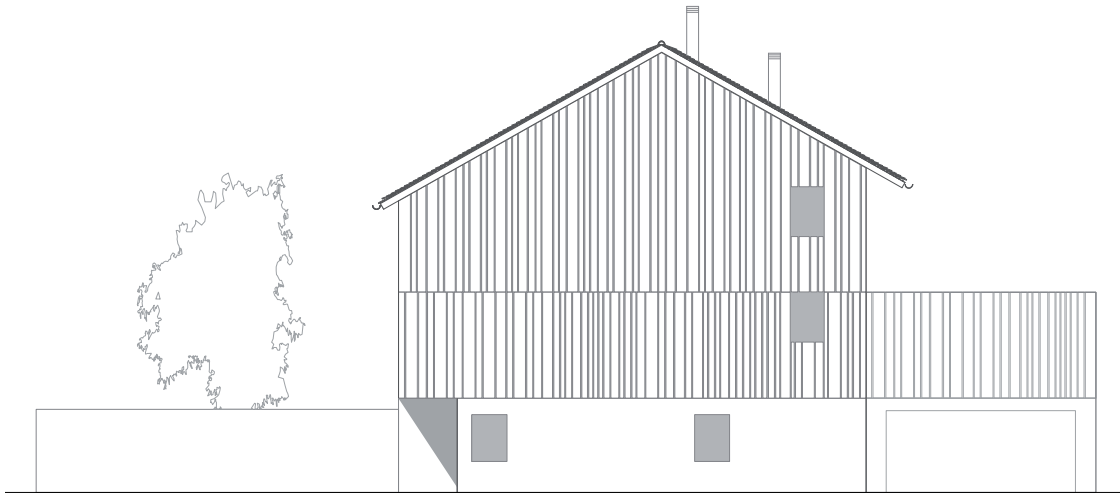
élévation nord
