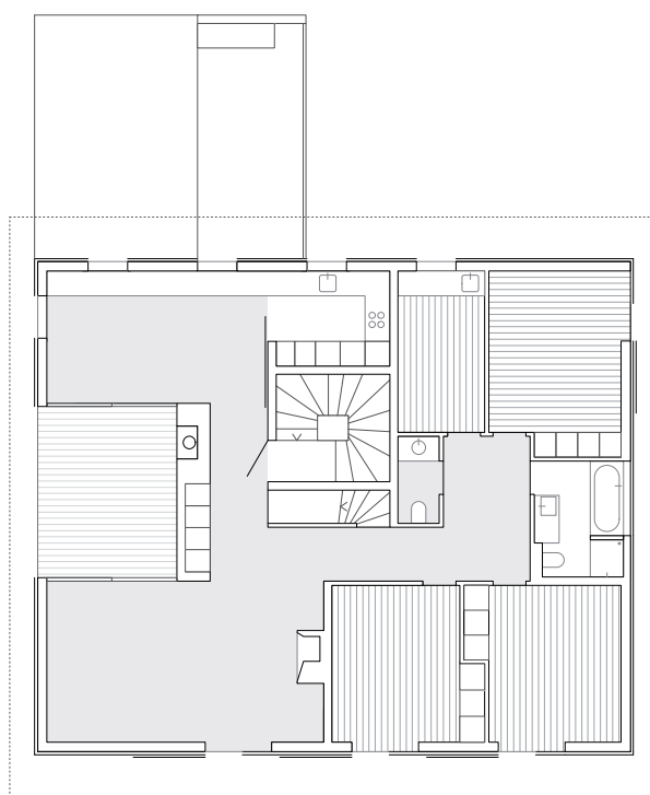
2ème étage
