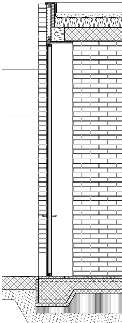
Coupe B
