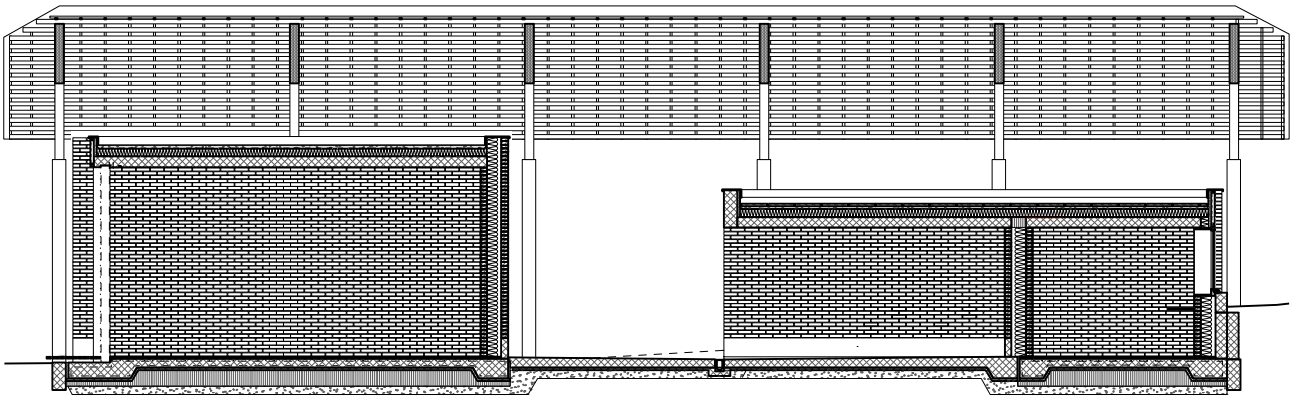
Coupe A
