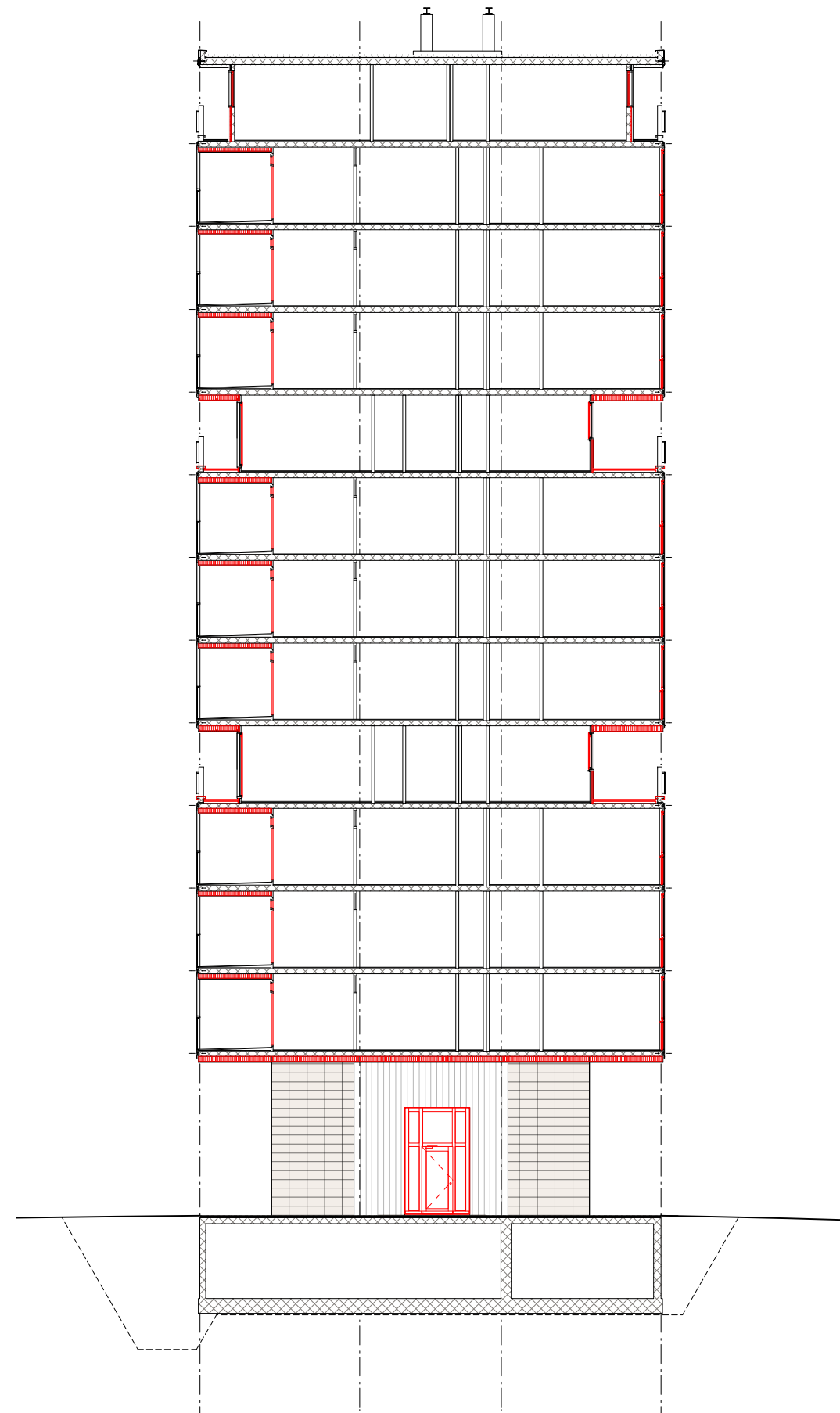
Façade et coupe de deux immeubles types
