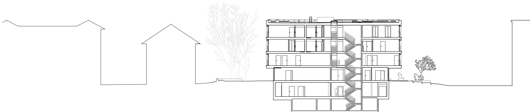
coupe transversale
