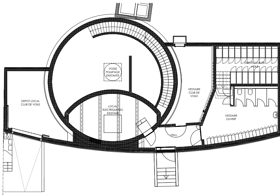
Plan du sous-sol
