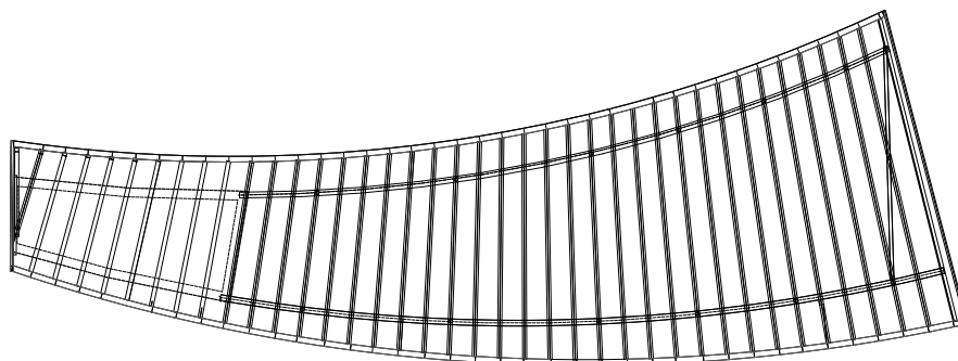
Plan de toiture
