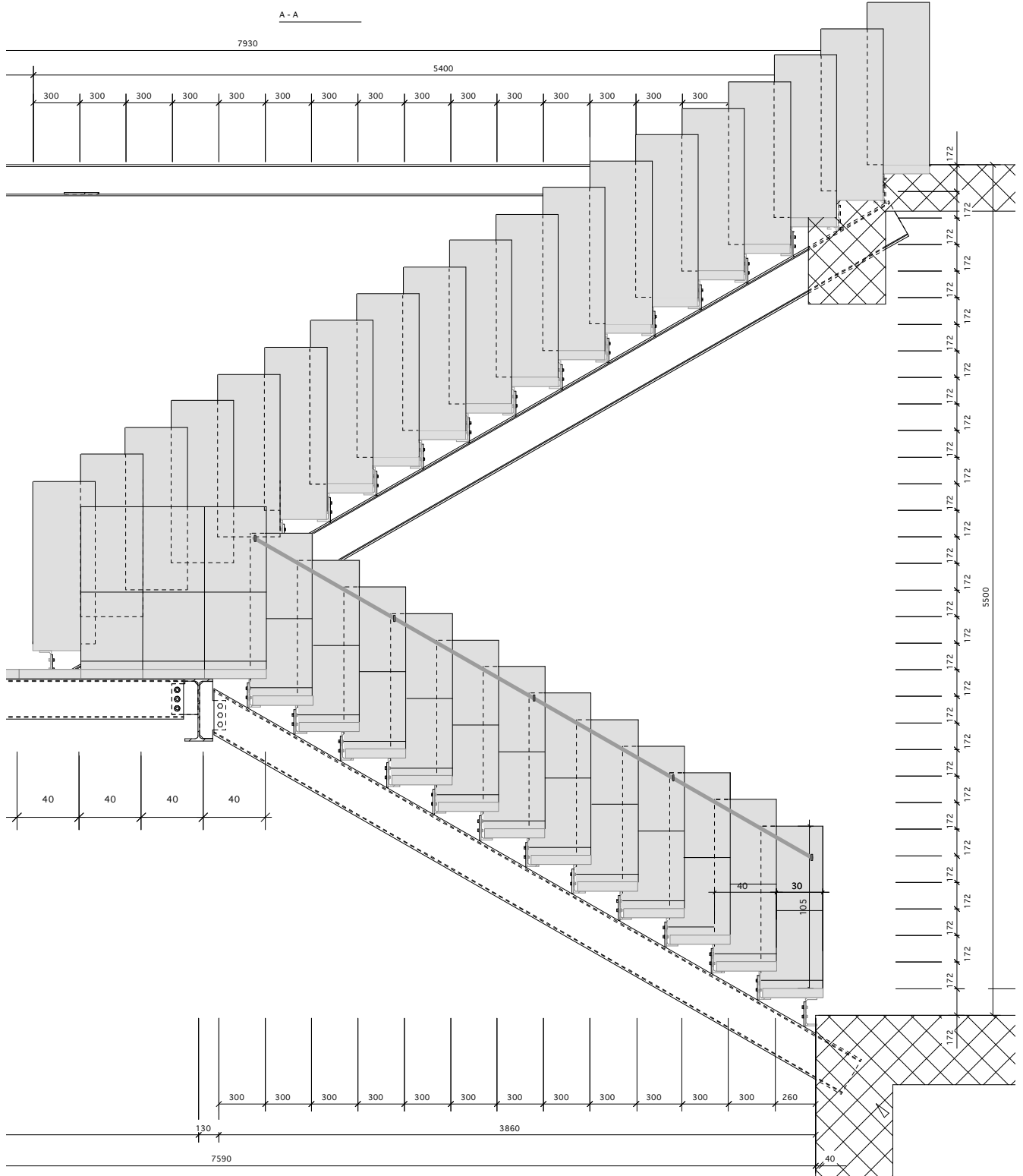
Coupe détail
