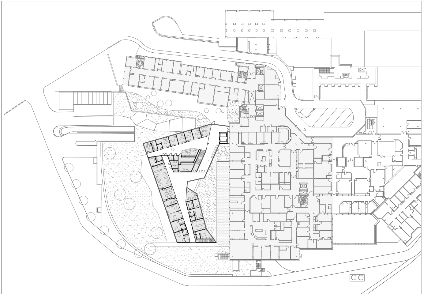
plan supérieur 1/1000
